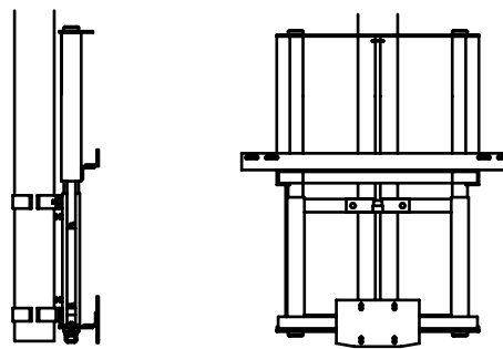
Fan Bank Manual Height Adjuster
